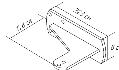
Кронштейн привода на столб
