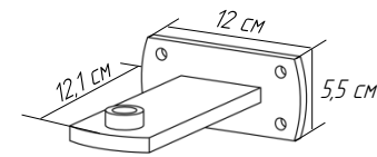
Кронштейн привода на створку
